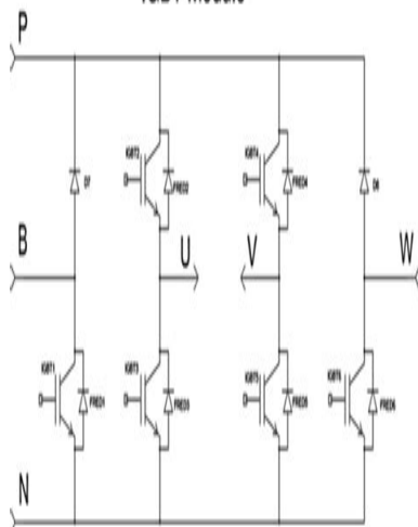
IGBT Module
